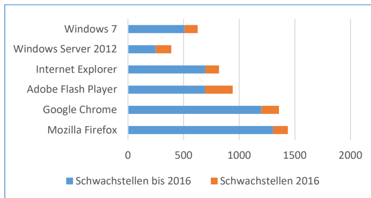
Schwachstellenüberblick 2 verschiedener Software-Produkte
