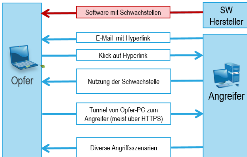
Mögliches Angriffsszenario durch eine Software-Schwachstelle
